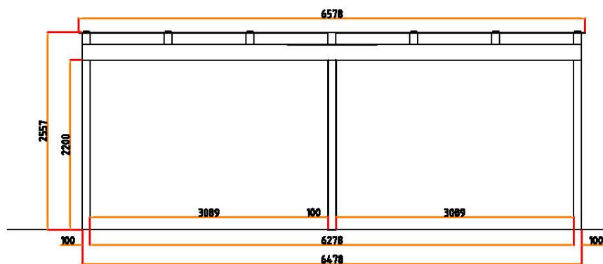
Čelní pohled
