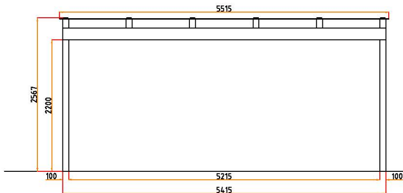
Čelní pohled
