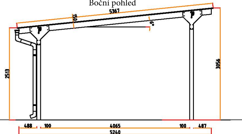
Boční pohled
