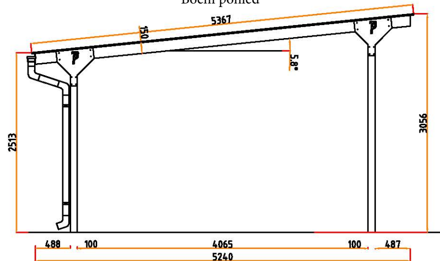
Boční pohled
