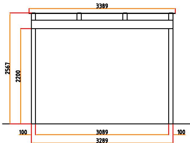
Čelní pohled
